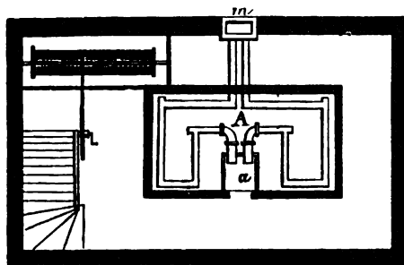
Fig. 363.—Ground-plan of kiln.
